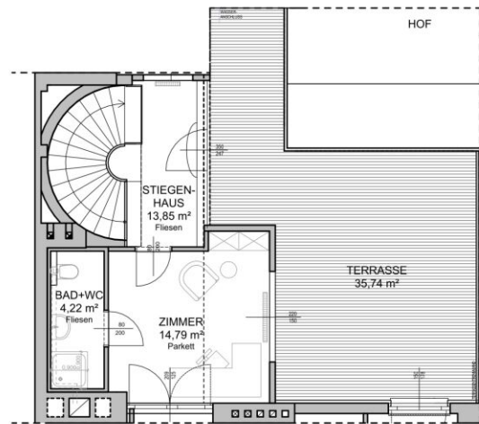
2. DACHGESCHOSS
